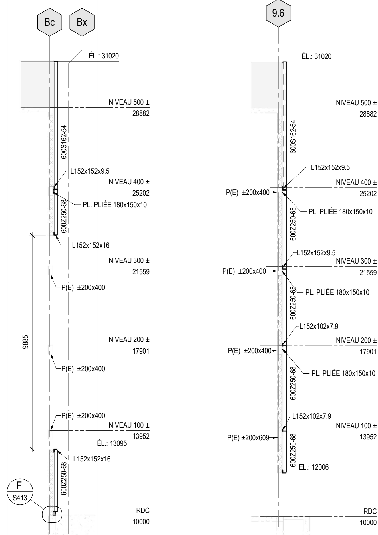
5 COUPE ESCALIER #3 S413 1:100
