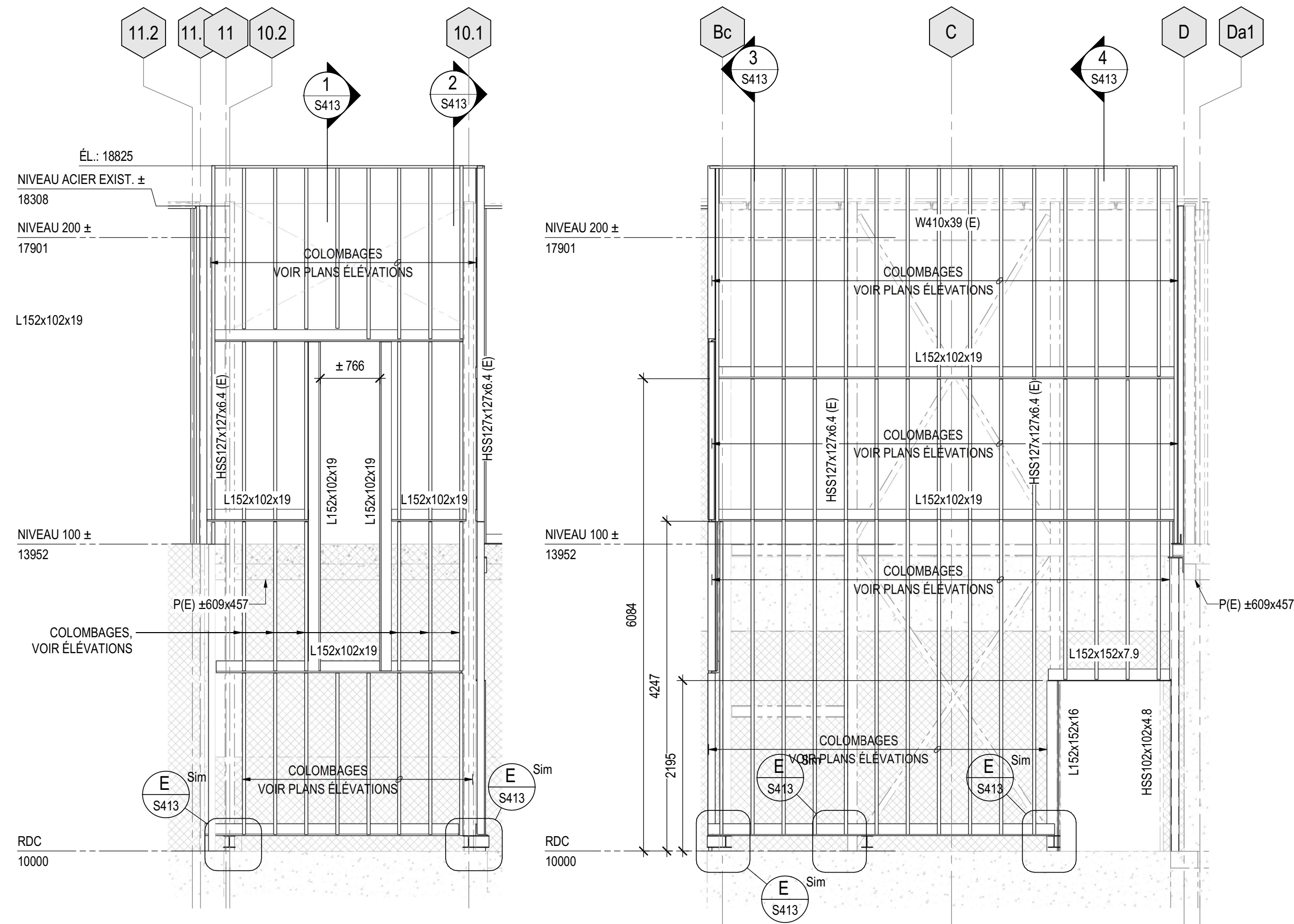
A ÉLEVATION ESCALIER #6 S302 1:50
