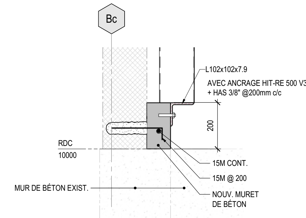
E DÉTAIL CONNEXION À LA BASE D'ESCALIER #6 S413 1:10
