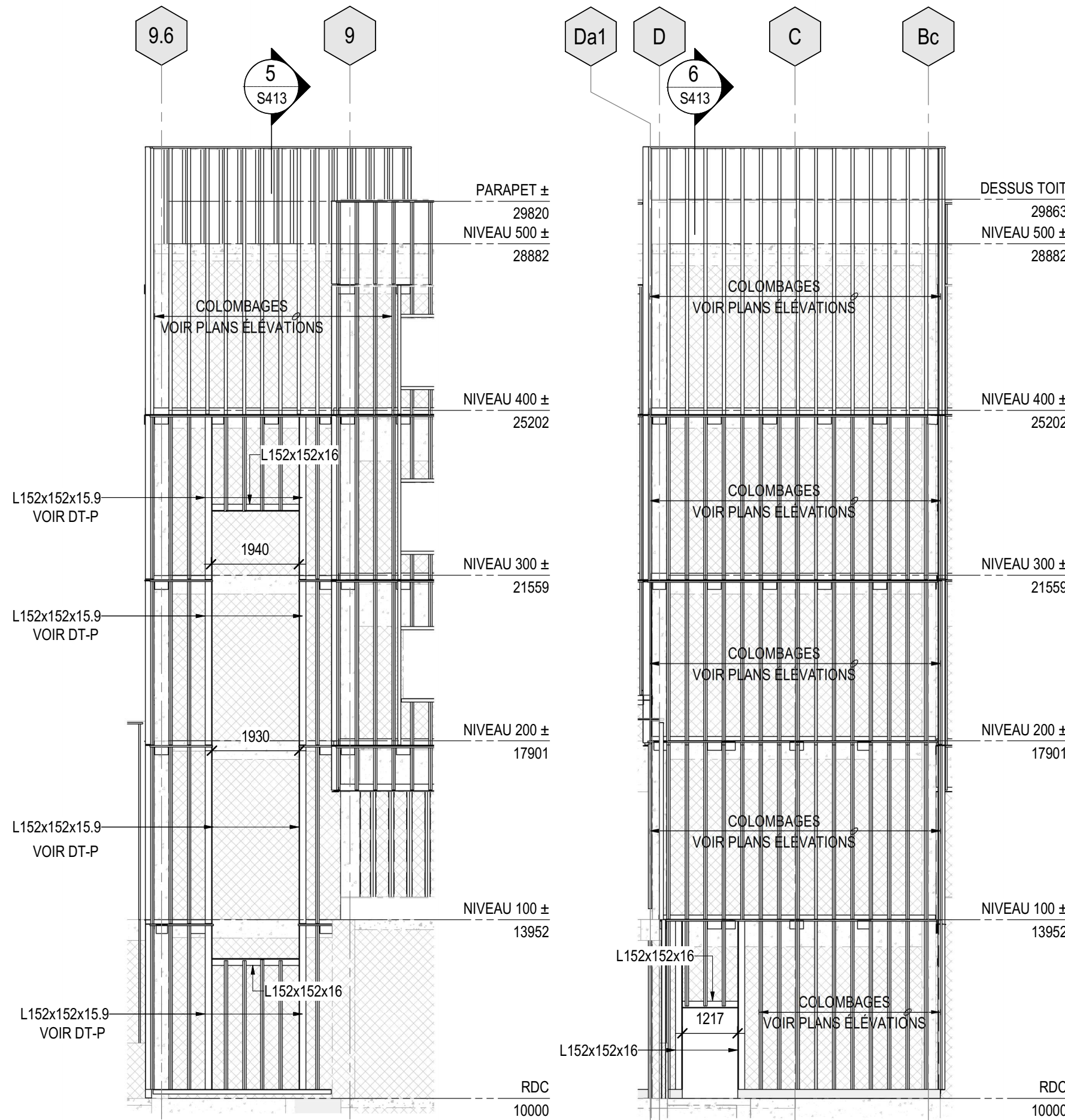
C ÉLEVATION ESCALIER #3 S302 1:100
