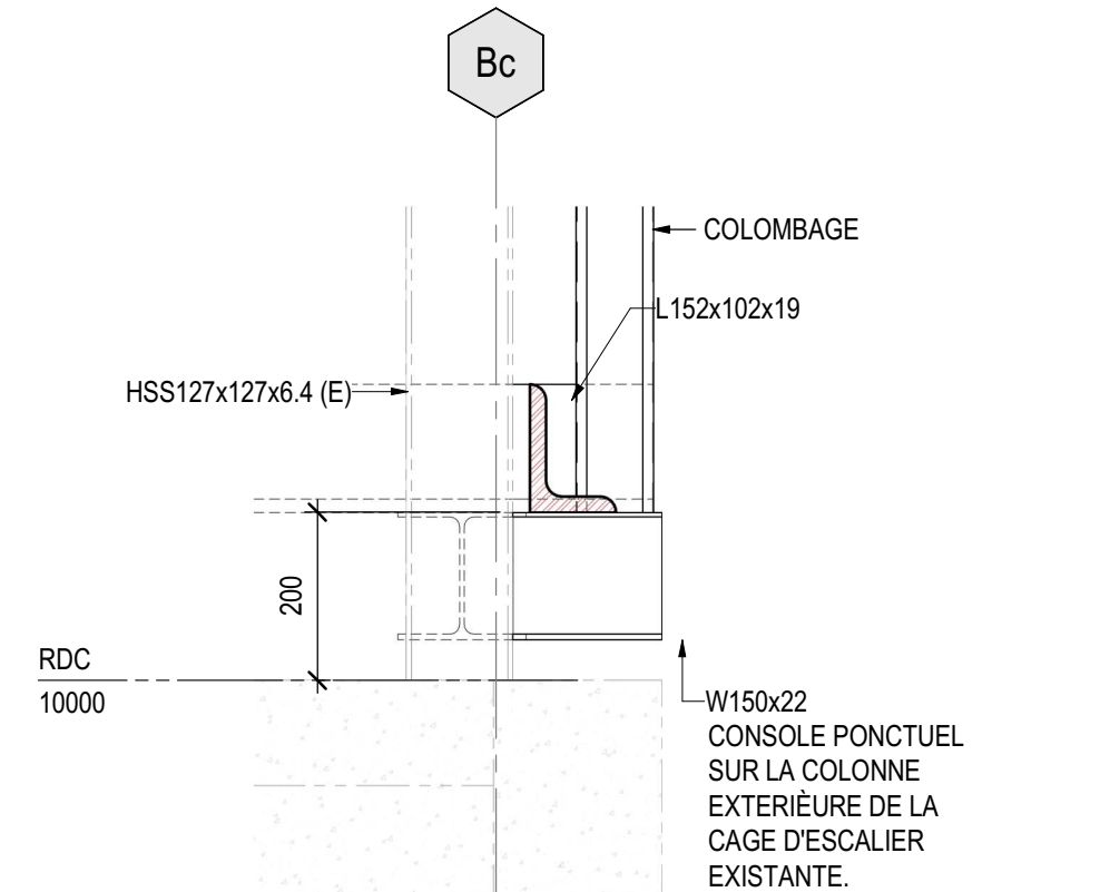
2 COUPE ESCALIER #6 S413 1:50
